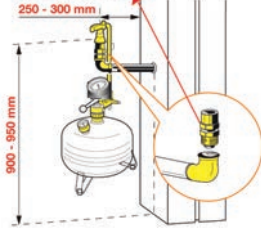
LATAUSASEMA Art. 52020 Sisältää Art. 52013
